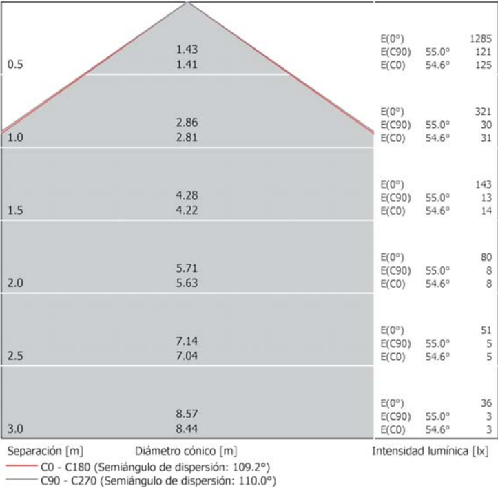
Diagrama Cónico
